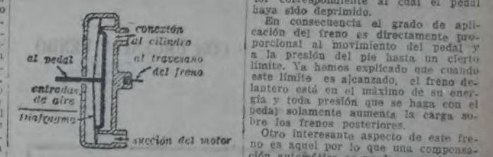
Fig. 3. — Válvula de control, reguladora de la succión del motor y del vacío en el cilindro.
